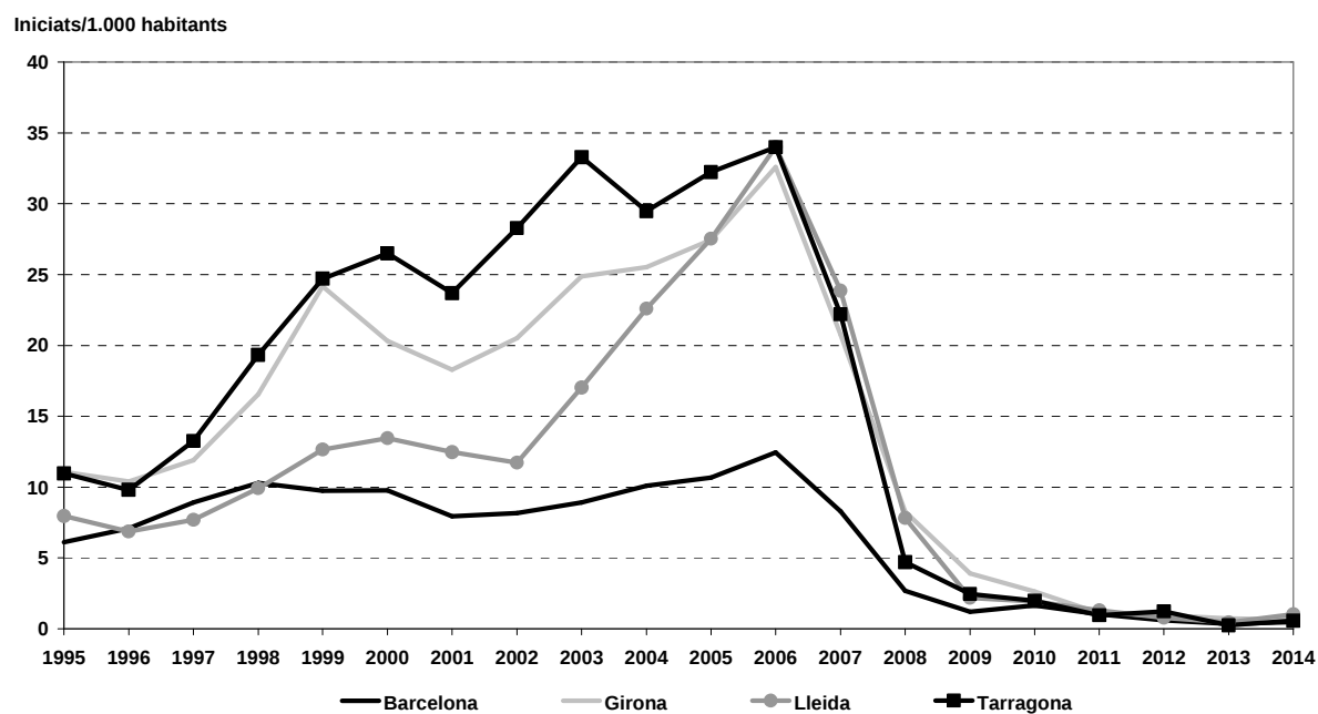
Gràfic 1.3 Evolució de la intensitat de la construcció d'habitatges per demarcacions territorials. 1995-2014
